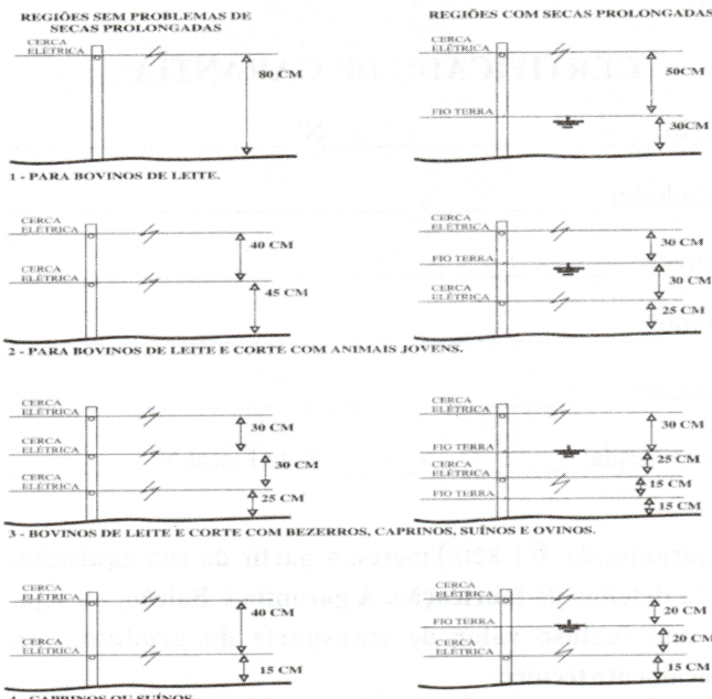
DISPOSIÇÃO DOS FIOS NA CERCA ELÉTRICA, CONSIDERANDO A ESPÉCIE ANIMAL E A CONDUTIVIDADE DO SOLO
